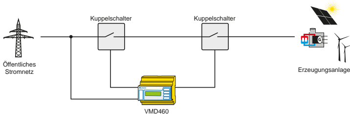
Abb. 4.1: Prinzipdarstellung eines zentralen NA-Schutzes mit Kuppelschaltern
