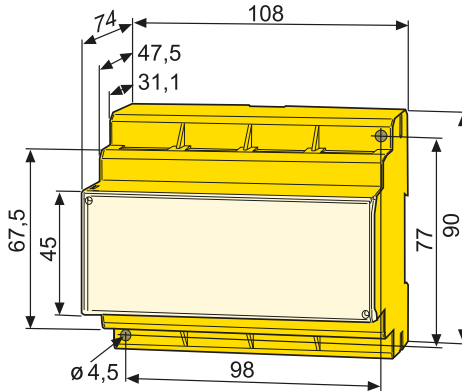
Abb. 4.2: Maßbild, Skizze für Schraubbefestigung
