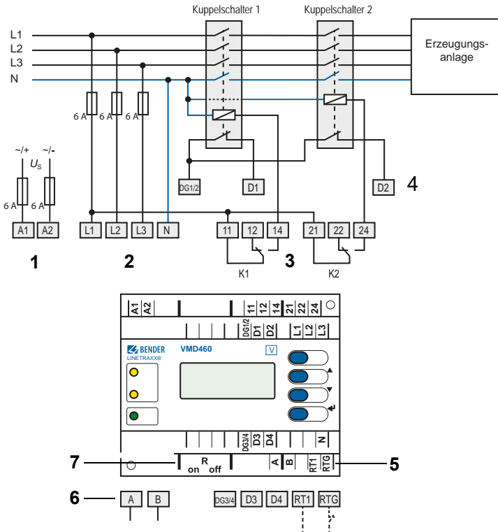
Abb. 4.3: Anschlussbild VMD460-NA (Normen 4105_1, 4105_2, 4110, BDEW, 0126, C10/11, G59/2, G59/3, G83/2, G98, G99)
