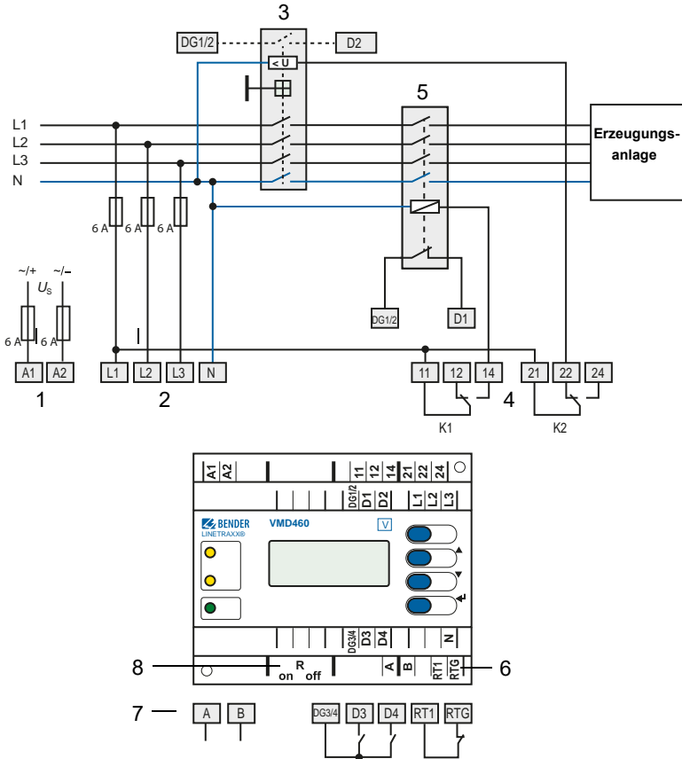
Abb. 4.4: Anschlussbild VMD460-NA (CEI 0-21)
