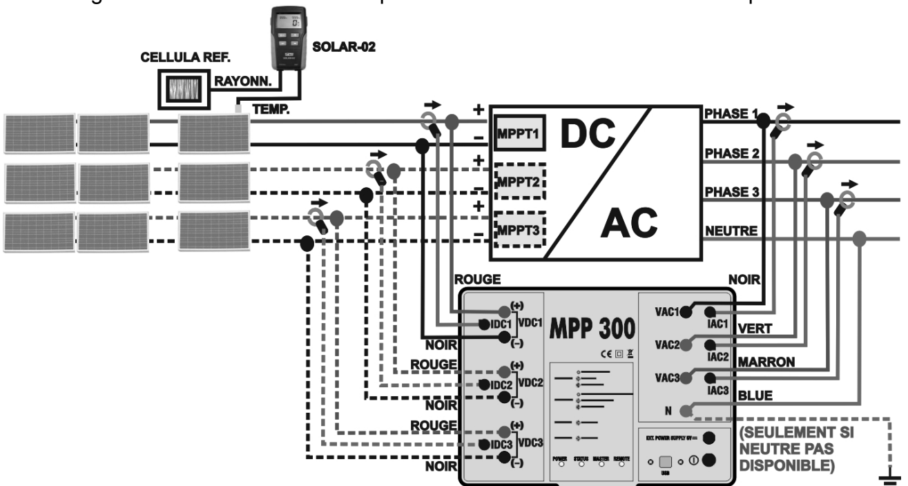
Fig. 6 : Connexion du MPP300 pour essai d'une installation PV Triphasée
