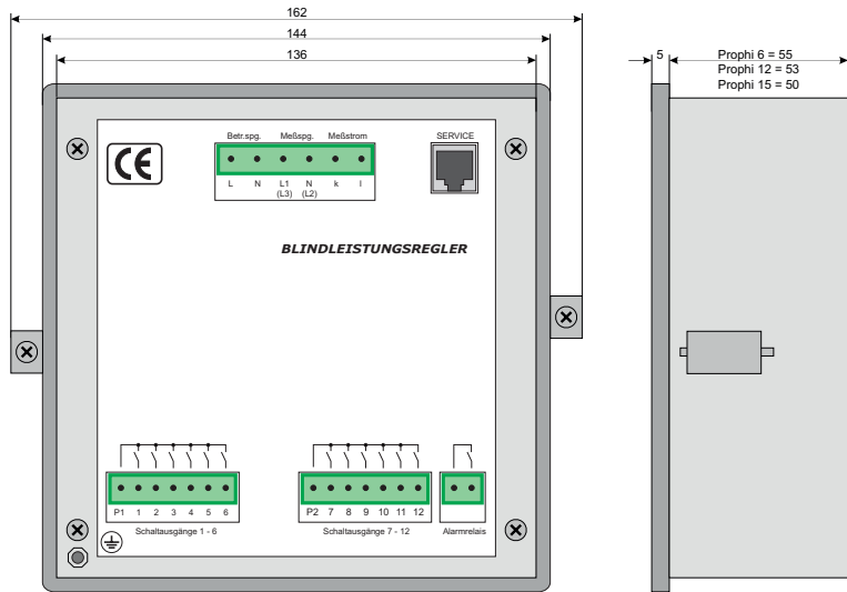
Ansicht Rückseite
