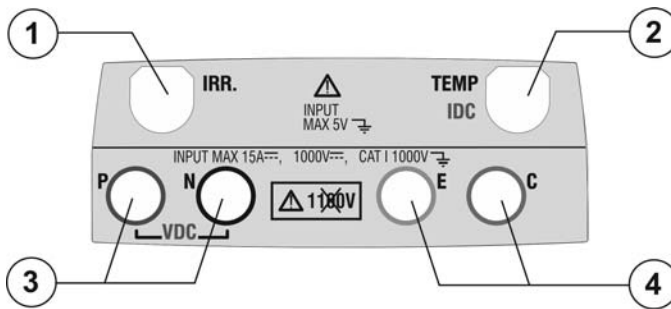
Abb. 2: Obenansicht
