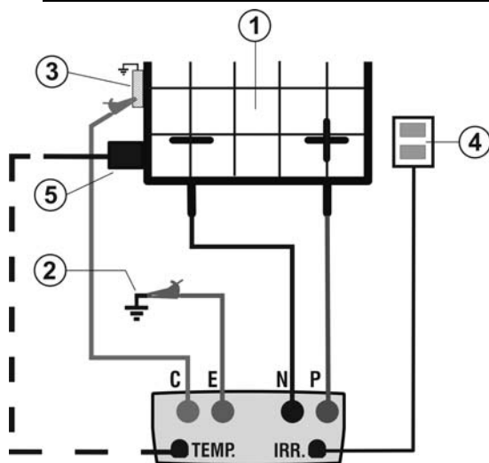
Abb. 8: Verbindung für IVCK Test mit direkter Einstrahlungsmessung
