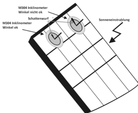
Abb. 7: Positionierung des optionalen Inclinometers M304
