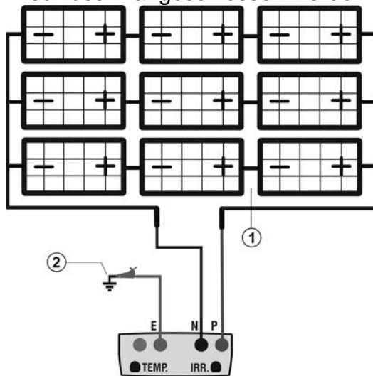
Abb. 10: Verbindung des Gerätes für Isolationmessung Betriebsmodus Feld -
