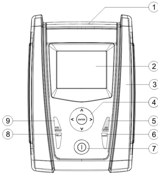
Abb. 1: Frontansicht
