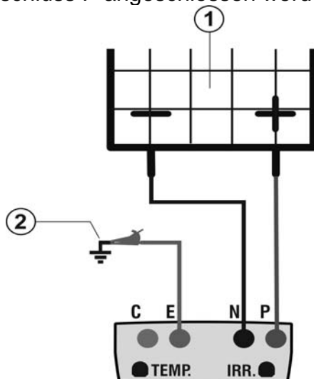
Abb. 12: Verbindung des Gerätes für Isolationsmessung - Betriebsmodus STRING
