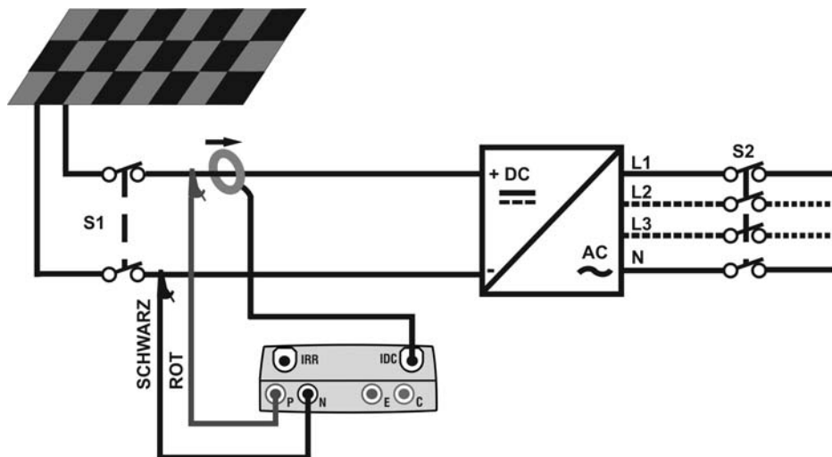
Abb. 5: Anschlussschema der Parameter einer PV-Anlage ohne SOLAR-02
