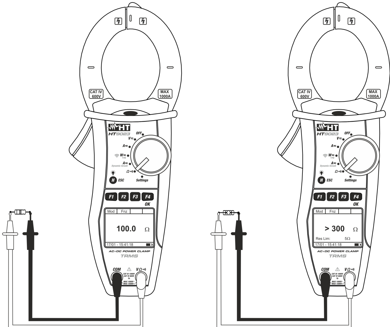
Abb. 14: Widerstandsmessung
