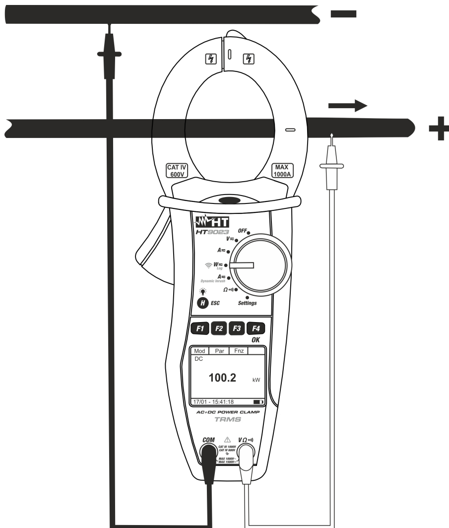
Abb. 12: DC Leistungsmessung
