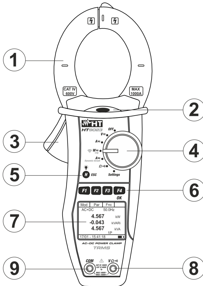
Abb. 1: Gerätebeschreibung
