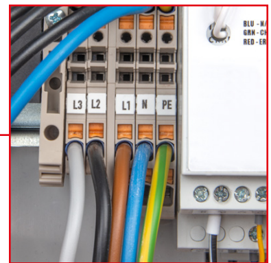
Anschluss 3-phasige Zuleitung (L3, L2, L1, N, PE)
