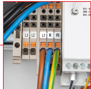
Anschluss 1-phasige Zuleitung (L1, N, PE)
