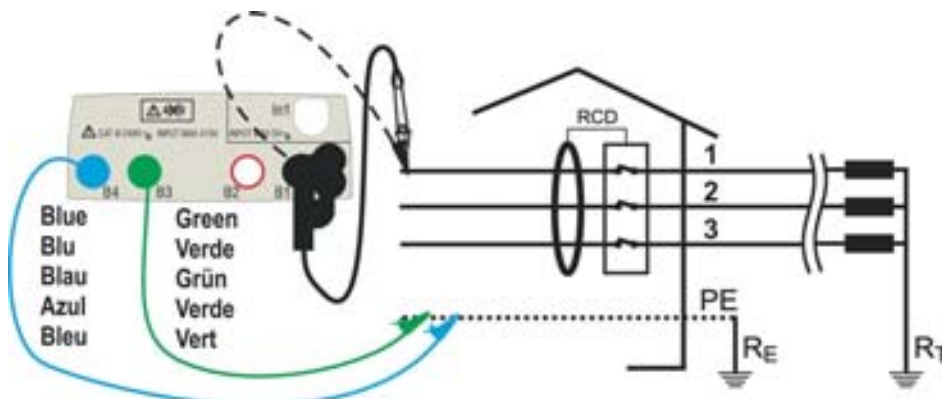
Fig. 16: Collegamento in sistema trifase 400V+ PE (no N) con cavi singoli e puntale remoto (no RCD tipo B)
