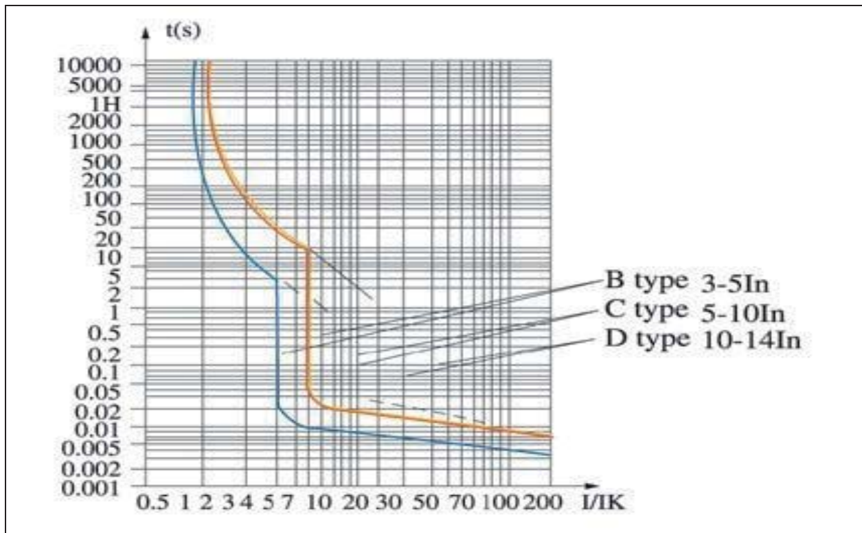
Fig. 45: Esempio di curve di intervento protezioni magnetotermiche (MCB)
