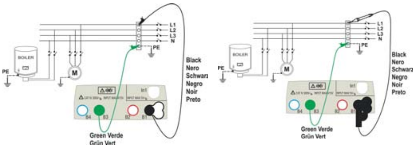
Fig. 8: Verifica dell'isolamento L-PE tramite cavi singoli e puntale remoto
