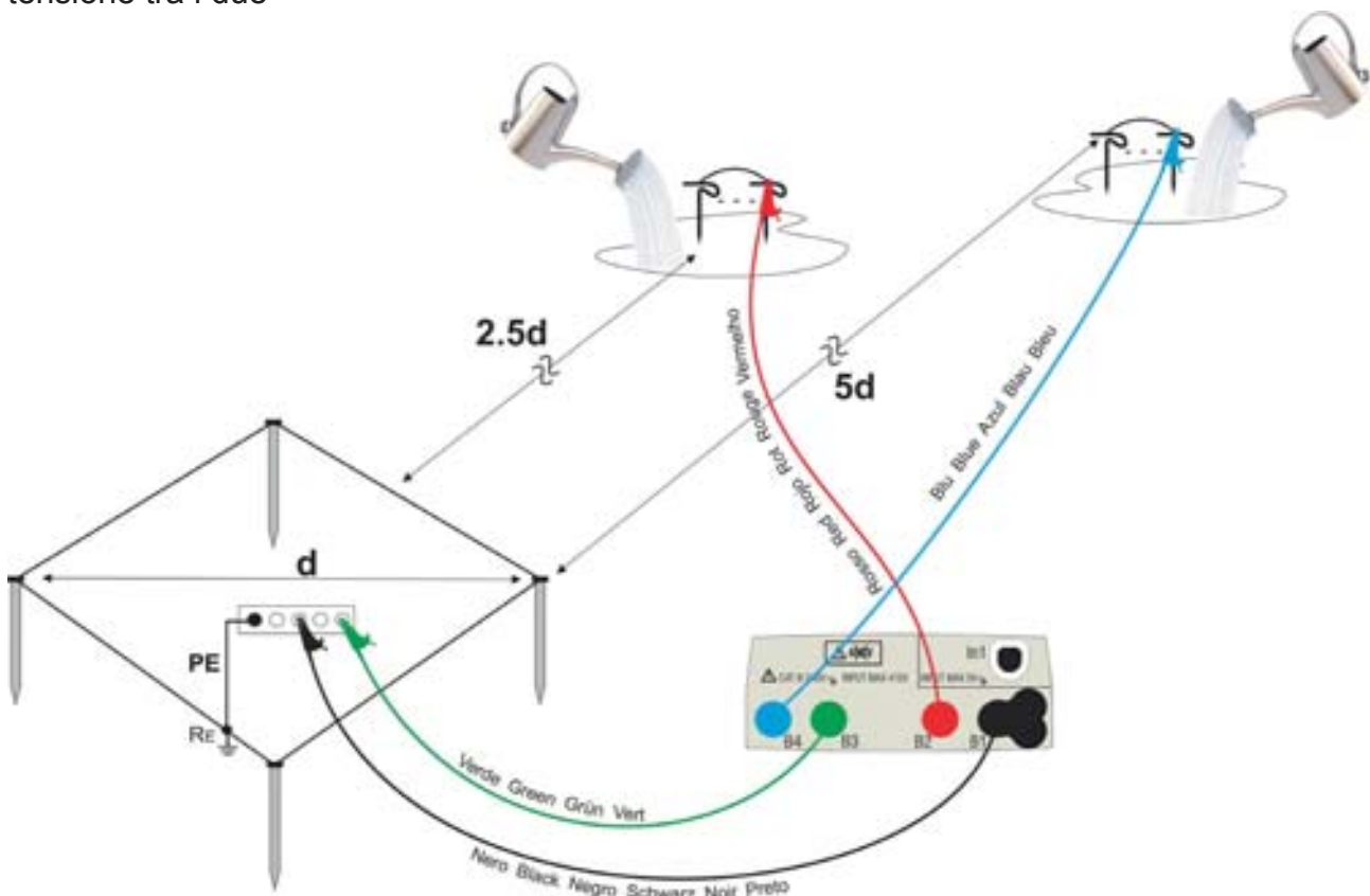
Fig. 46: Misura di terra per reti di terra di piccole dimensioni
