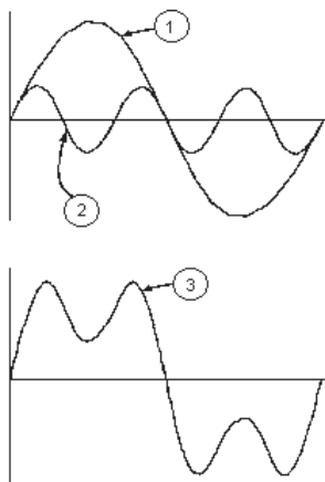
Fig. 50: Effetto della sovrapposizione di due frequenze multiple l'una dell'altra
