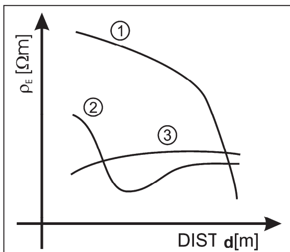
Fig. 49: Misura della resistività del terreno
