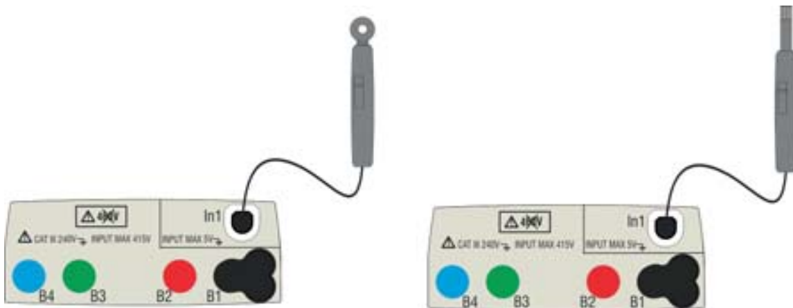
Fig. 33: Misura parametri ambientali con sonde esterne
