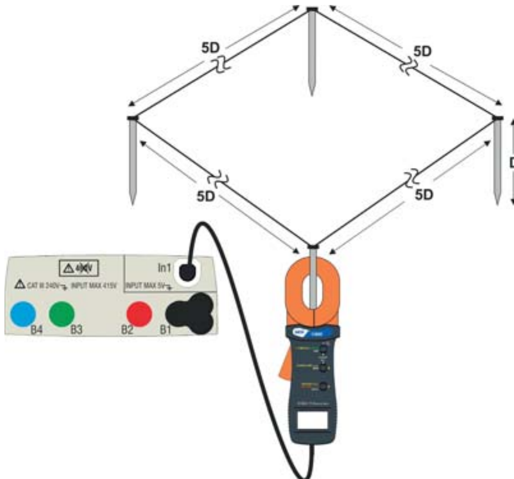
Fig. 32: Misura resistenza dispersori singoli con pinza T2100
