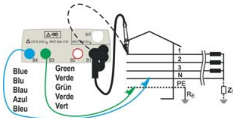
Fig. 23: Misura P-PE in sistemi IT con cavi singoli e puntale remoto
