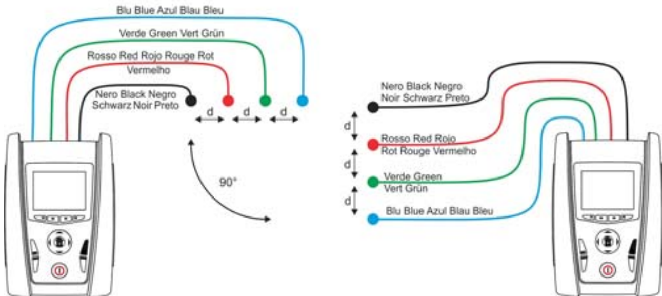
Fig. 48: Misura della resistività del terreno
