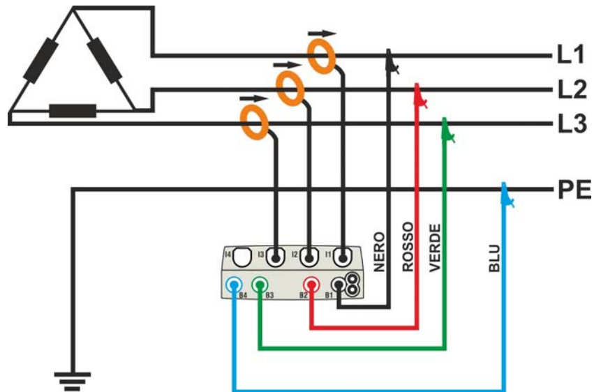
Fig. 38: Collegamento per misura su impianto Trifase 3\phi -ARON
