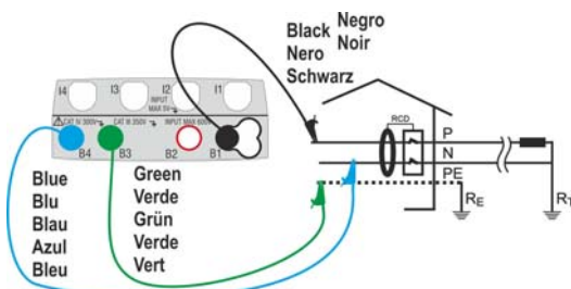
Fig. 12: Collegamento in sistema monofase 230V con cavi singoli e puntale remoto
