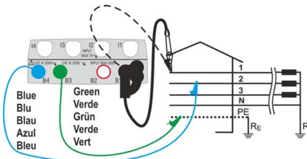
Fig. 20: Misura P-P in impianti trifase 400V + N + PE
