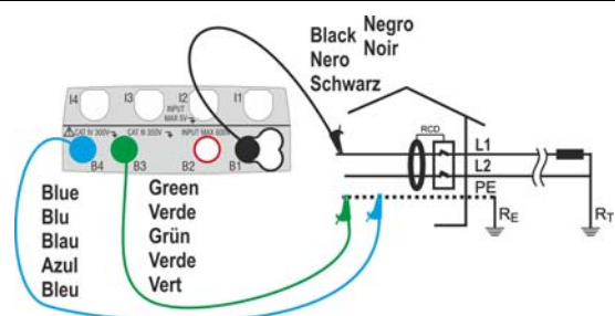
Fig. 11: Collegamento in sistema bifase 230V senza neutro (no RCD tipo B)
