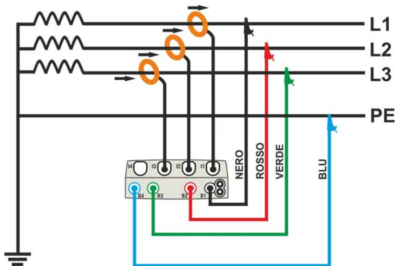
Fig. 37: Collegamento per misura su impianto Trifase 3φ-3FILI
