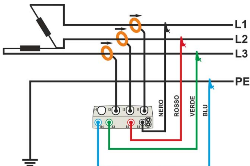
Fig. 40: Collegamento per misura su impianto Trifase 3\phi - \Delta Aperto – sistemi USA
