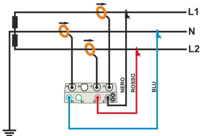
Fig. 43: Collegamento per misura su impianto Bifase 1\phi -PresaCentrale – sistemi USA
