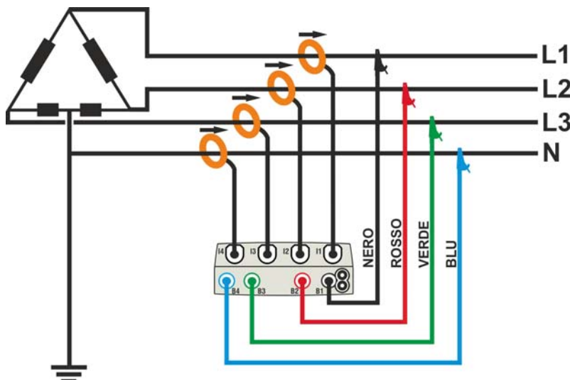
Fig. 39: Collegamento per misura su impianto Trifase 3\phi -High Leg – sistemi USA
