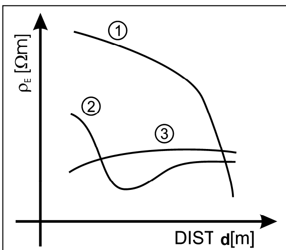
Fig. 50: Misura della resistività del terreno
