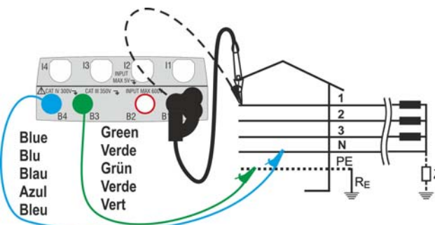
Fig. 22: Misura P-PE in sistemi IT con cavi singoli e puntale remoto
