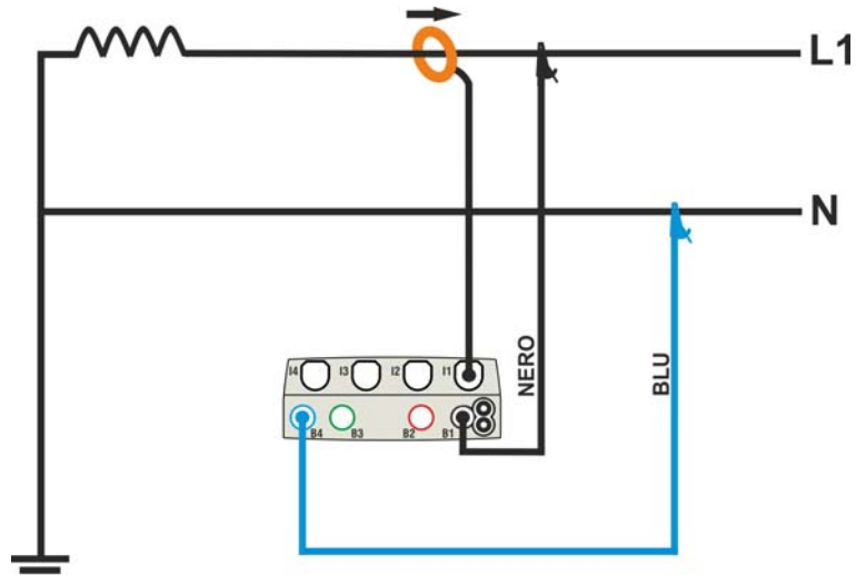
Fig. 35: Collegamento per misura su impianto Monofase 1φ-2FILI
