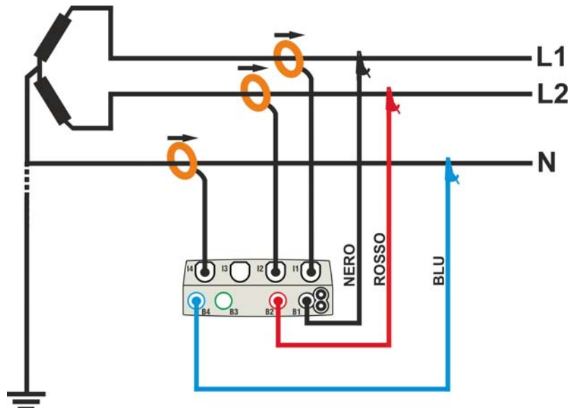
Fig. 41: Collegamento per misura su impianto Bifase 3\phi -Y Aperta – sistemi USA
