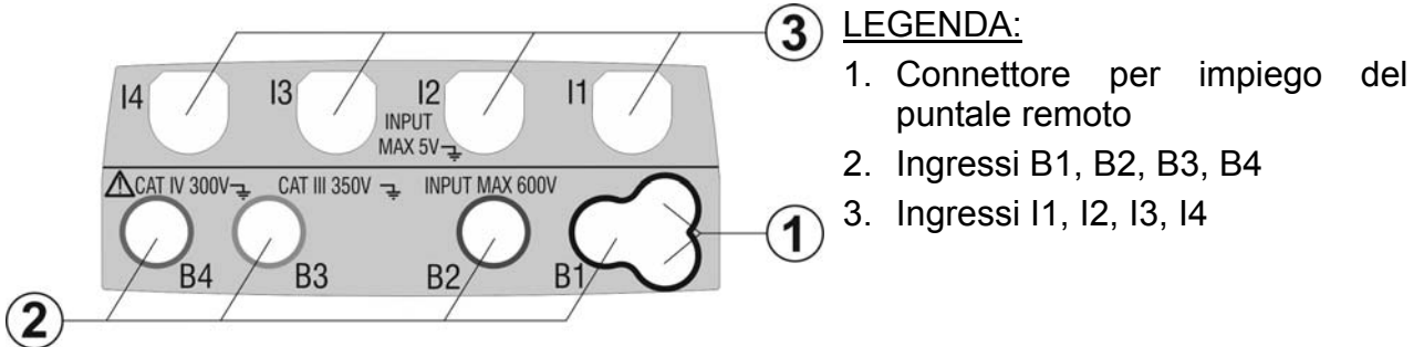
Fig. 2: Descrizione parte superiore dello strumento
