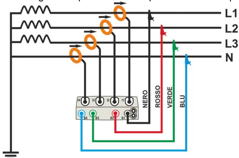
Fig. 36: Collegamento per misura su impianto Trifase 3φ-4FILI
