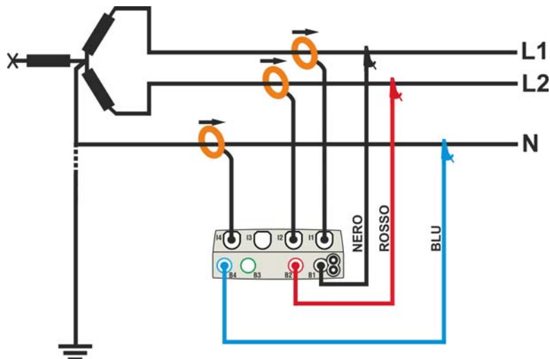
Fig. 42: Collegamento per misura su impianto Bifase 3\phi -2EI. \frac{1}{2} – sistemi USA
