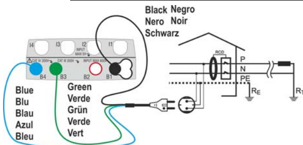
Fig. 10: Collegamento in sistema monofase 230V tramite spina shuko
