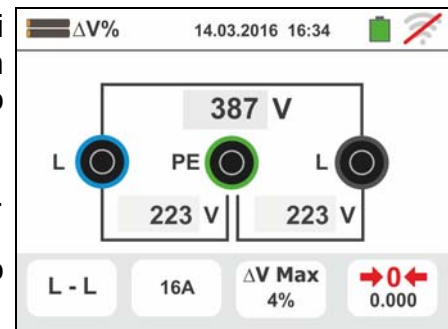
Fig. 34: Collegamento strumento per misura caduta di tensione in modo L-L
