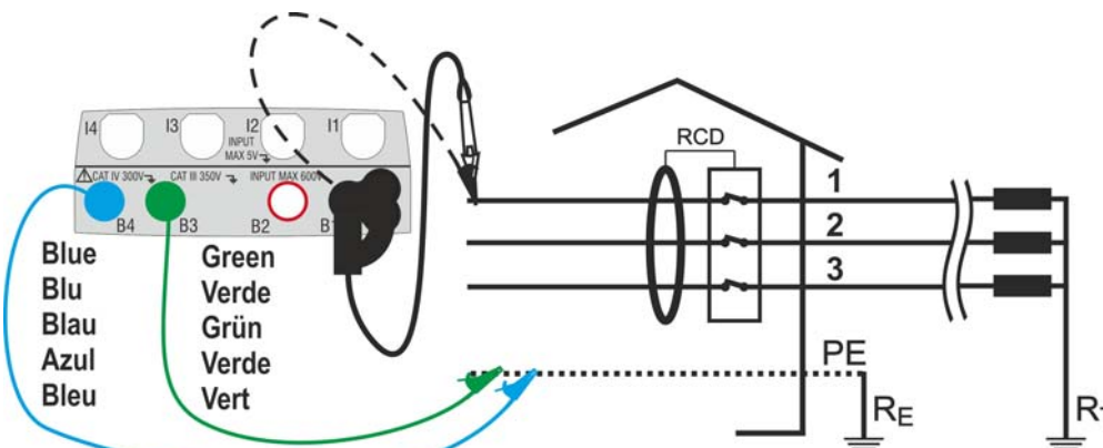
Fig. 15: Collegamento 400V+ PE (no N) con cavi e puntale remoto (no RCD tipo B)
