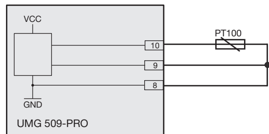
Abb. Schematische Darstellung des Anschlussbeispiels
