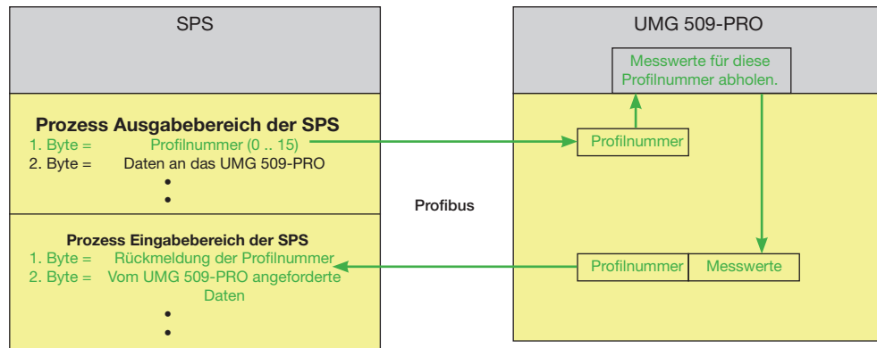
Abb. Blockschaltbild für den Datenaustausch zwischen SPS und UMG 509-PRO.
