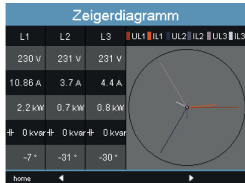
Abb. Zeigerdiagramm
