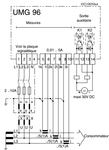
Fig.: Exemple de raccordement 3 Mesure 3 fils avec transformateurs d'intensité et trois transformateurs d'intensité.
