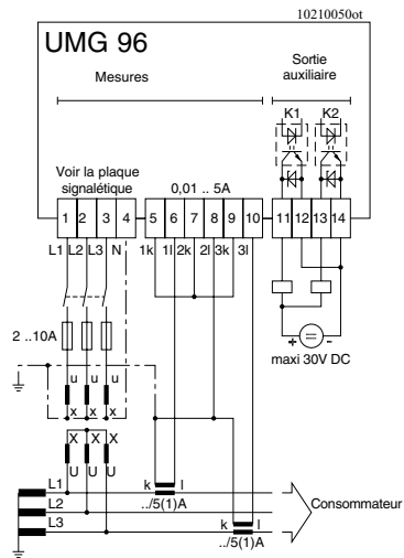
Fig.: Exemple de raccordement 4 Mesure 3 fils avec transformateurs d'intensité et deux transformateurs d'intensité.
