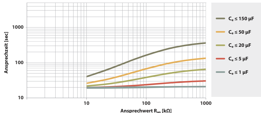
Ansprechzeit in Abhängigkeit vom Ansprechwert und der Netzableitkapazität nach IEC 61557-8 ( U_n = AC\ 690\ V , f_n = 60\ Hz )
