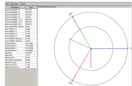
Abb.: GridVis® – Phasendiagramm
