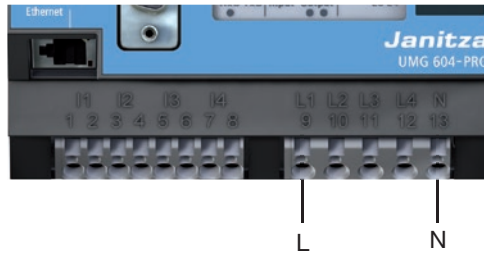
Abb. Spannungsmesseingangs mit angeschlossener Phase L und Neutralleiter N
