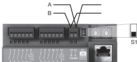
Fig.: Posizionamento a metà del segmento; terminazione via DIP switch S1 deattivata (OFF)
