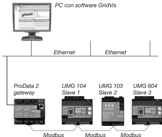
Fig.: Variante di connessione con il ProData 2 come gateway.
