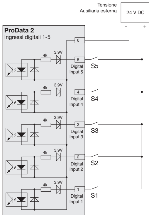
Fig. Esempio della connessione degli interruttori esterni dei contatti S1-S5 agli ingressi digitali 1-5.
