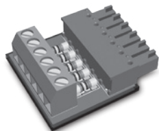
Fig.: Modulo S0 estraibile per connettere trasduttori di impulsi S0
