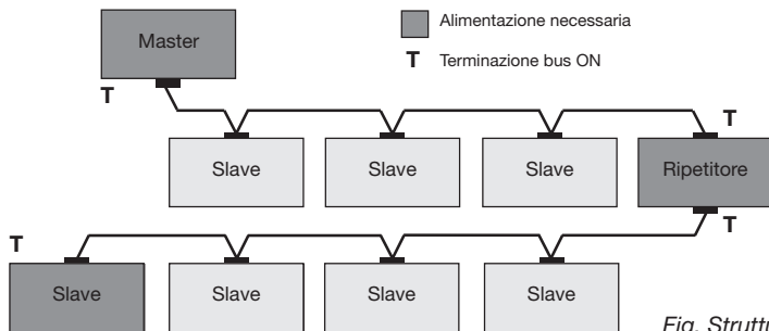
Fig. Struttura del bus
