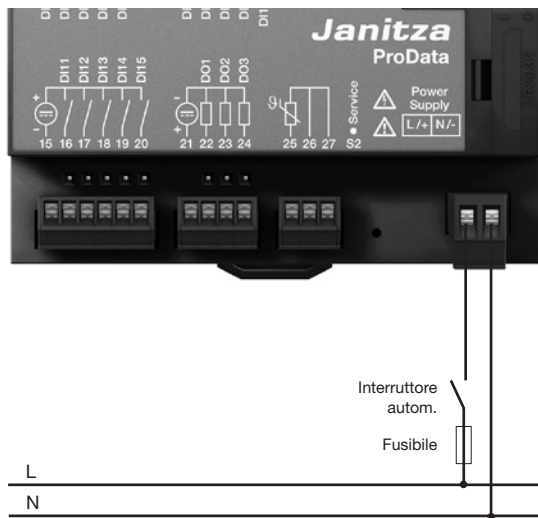
Fig. Esempio di connessione della tensione di alimentazione a un ProData 2.
