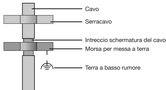
Fig. Procedura di schermatura all'entrata nell'armadio.
