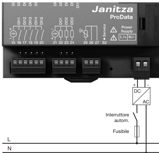
Fig. Esempio di connessione della tensione di alimentazione a un ProData 2 attraverso alimentazione esterna.
