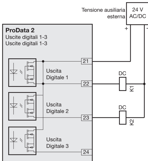
Fig. Esempio di due relè connessi alle uscite digitali
