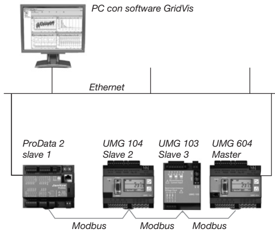
Fig.: Variante di connessione con il ProData 2 come dispositivo slave Modbus RTU.
