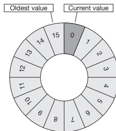
Fig.: Memoria ad anello per 16 elementi
