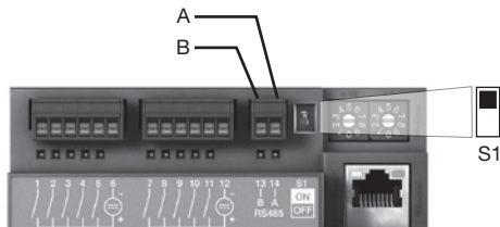
Fig.: Posizionamento alla fine del segmento; terminazione via DIP switch S1 attivata (ON)
