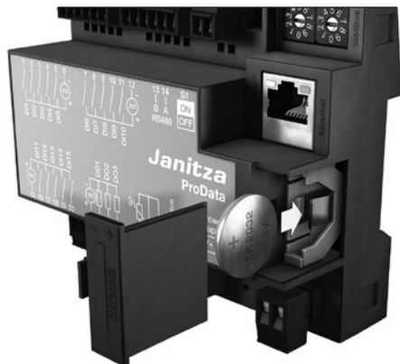
Fig. Compartimento per la batteria sul lato frontale
