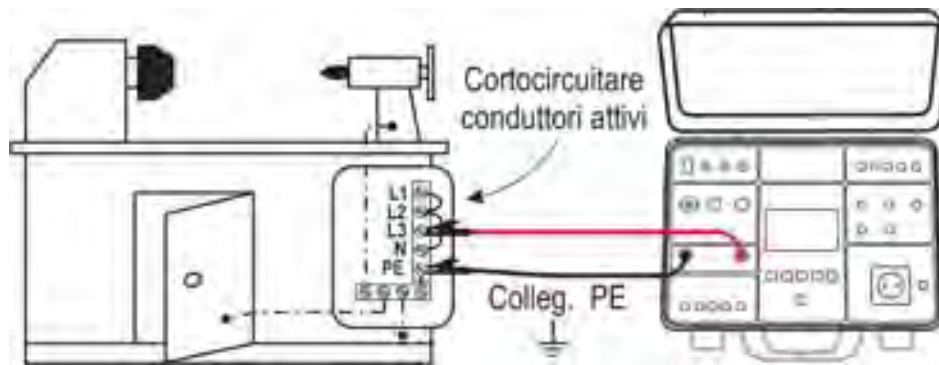
Fig. 33: Collegamento dei terminali per misura M\Omega
