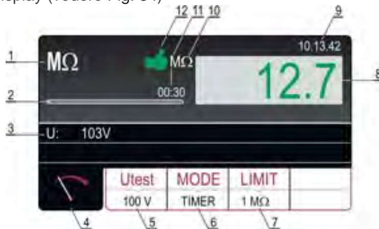
Fig. 34: Risultato misura M\Omega
