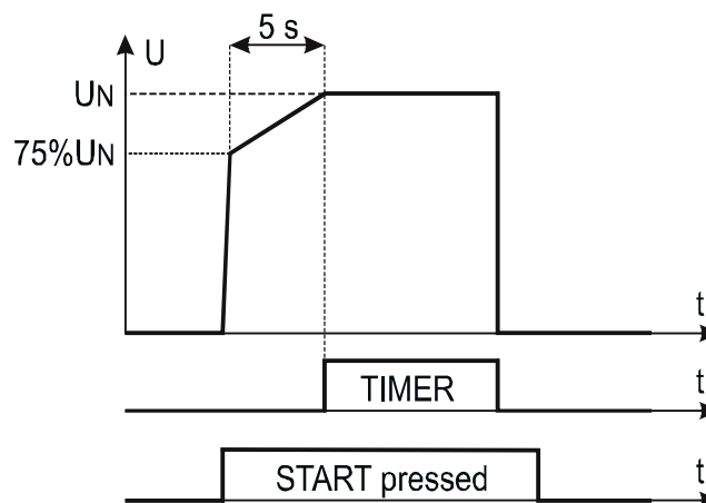
Fig. 37: Test Rigidità Dielettrica in modo Rampa 75%
